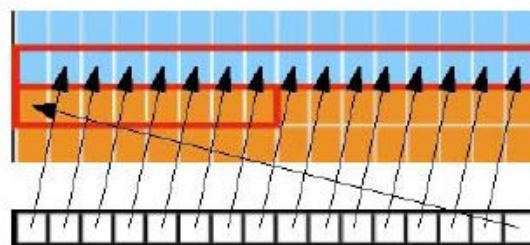
Figura 3 Ejemplo de 16 accesos que se agrupan en 2 accesos a memoria. (NVIDIA 2010b)
